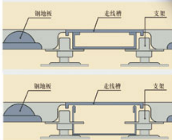
安装剖面图
